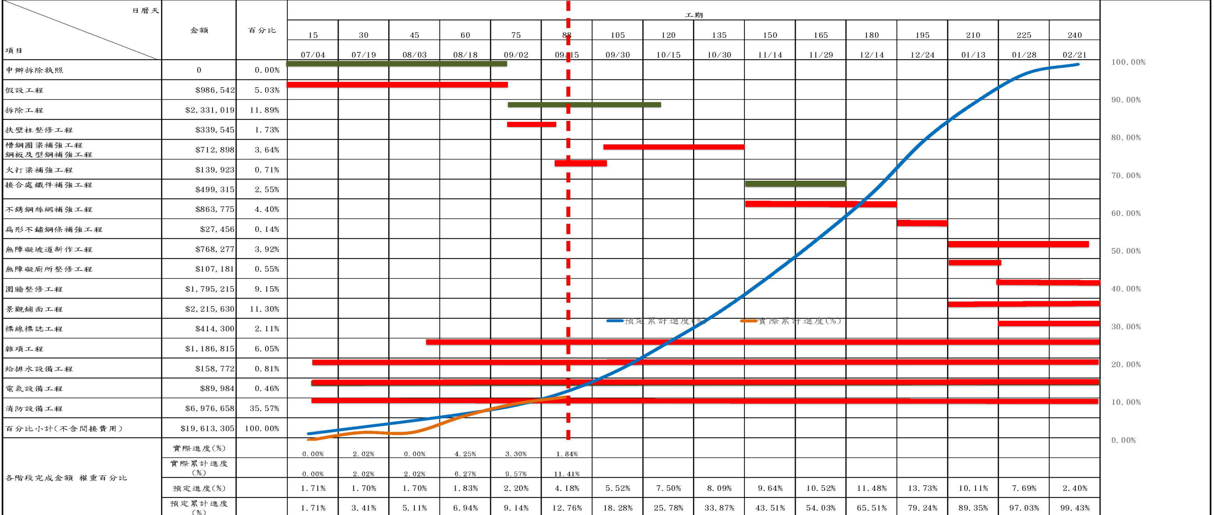
國定古蹟-嘉義舊監獄園區因應計畫改善工程預定進度甘特圖
