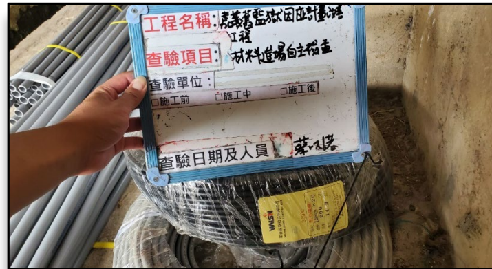
消防設備進場
