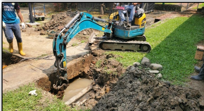
消防管溝開挖
