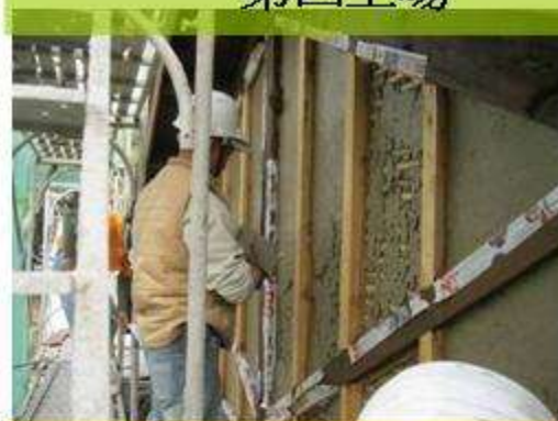
編竹夾泥牆施作
